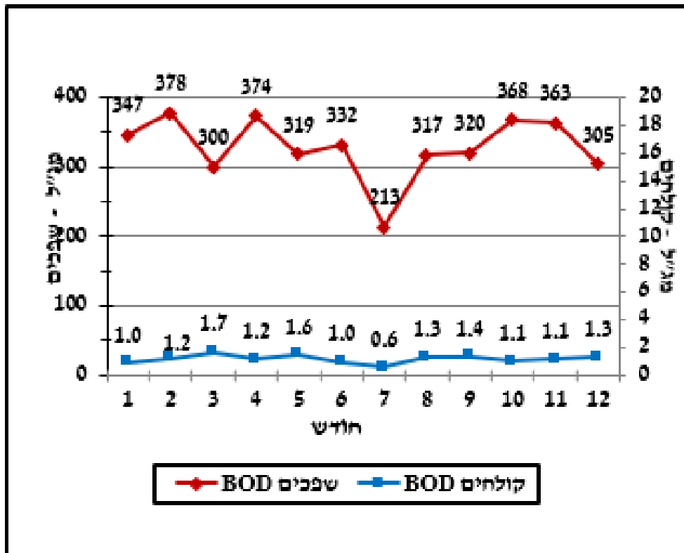
איור 8: ריכוזי צח"ב (BOD) בשפכים ובקולחים 2023
