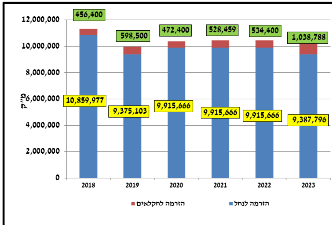
איור 3: פילוג שימוש שנתי בקולחים ממט"ש כפר סבא והוד השרון 2018-2023
