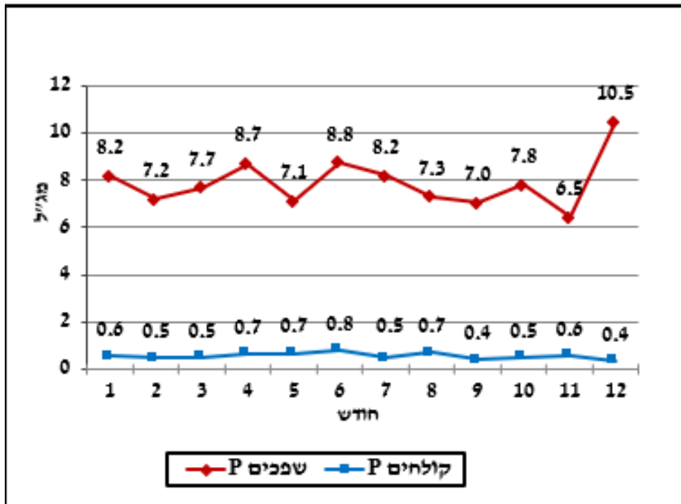
איור 11: ריכוזי זרחן (Pt) בשפכים הגולמיים ובקולחים 2023
