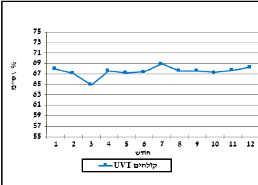
איור 14: ערכי UVT בקולחים 2023
