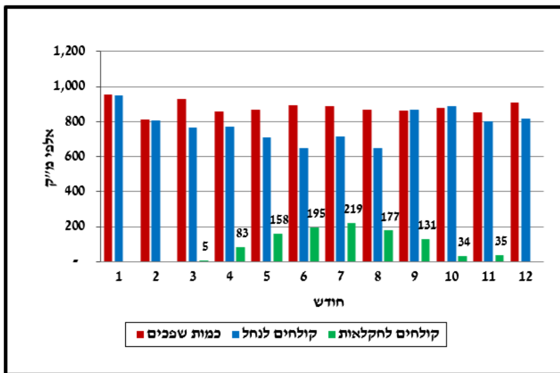
איור 4: ספיקת שפכים וקולחים לנחל ולחקלאות לפי חודשים בשנת 2023
