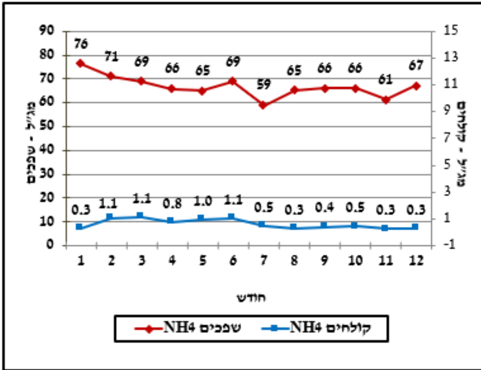
איור 12: ריכוז חנקן אמוניקלי בשפכים ובקולחים 2023
