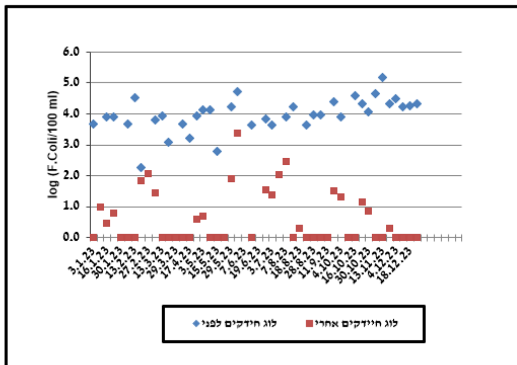
איור 16: ספירות חיידקי ק. צואתי בכניסה וביציאה מתעלת ה-UV (בלוג/100ml) (cfu)
