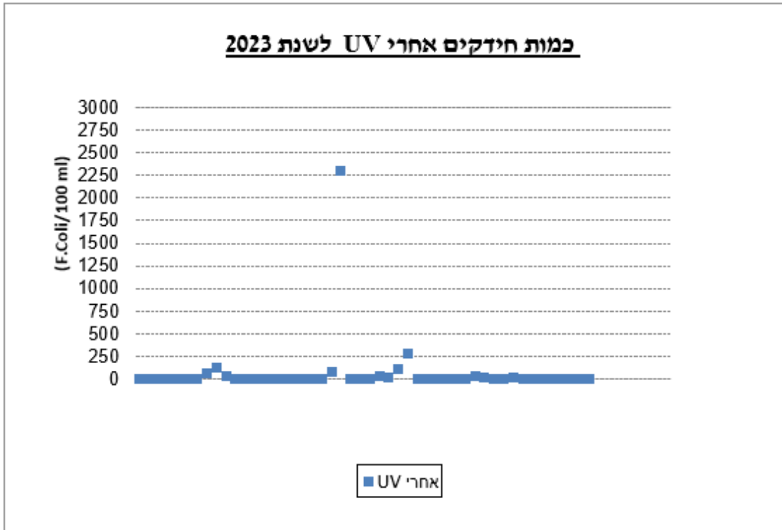
איור 17: כמות חיידקי ק. צואתי בקולחים לאחר חיטוי (cfu/100ml)
