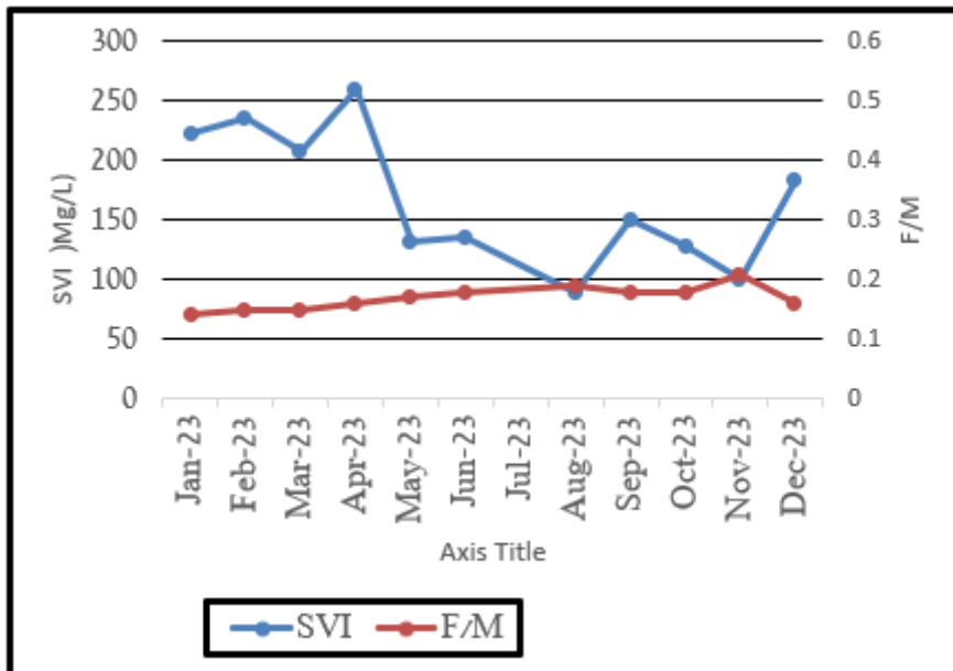
איור 6: מדד נפחיות הבוצה ויחס מזון/מיקרואורגניזמים
