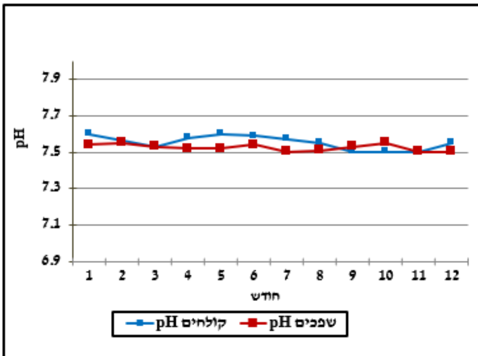
איור 13: pH בשפכים ובקולחים 2023
