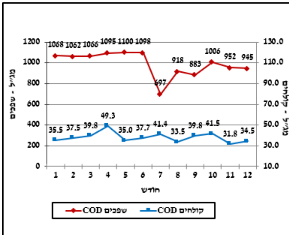
איור 9: ריכוזי צח"כ (COD) בשפכים ובקולחים 2023
