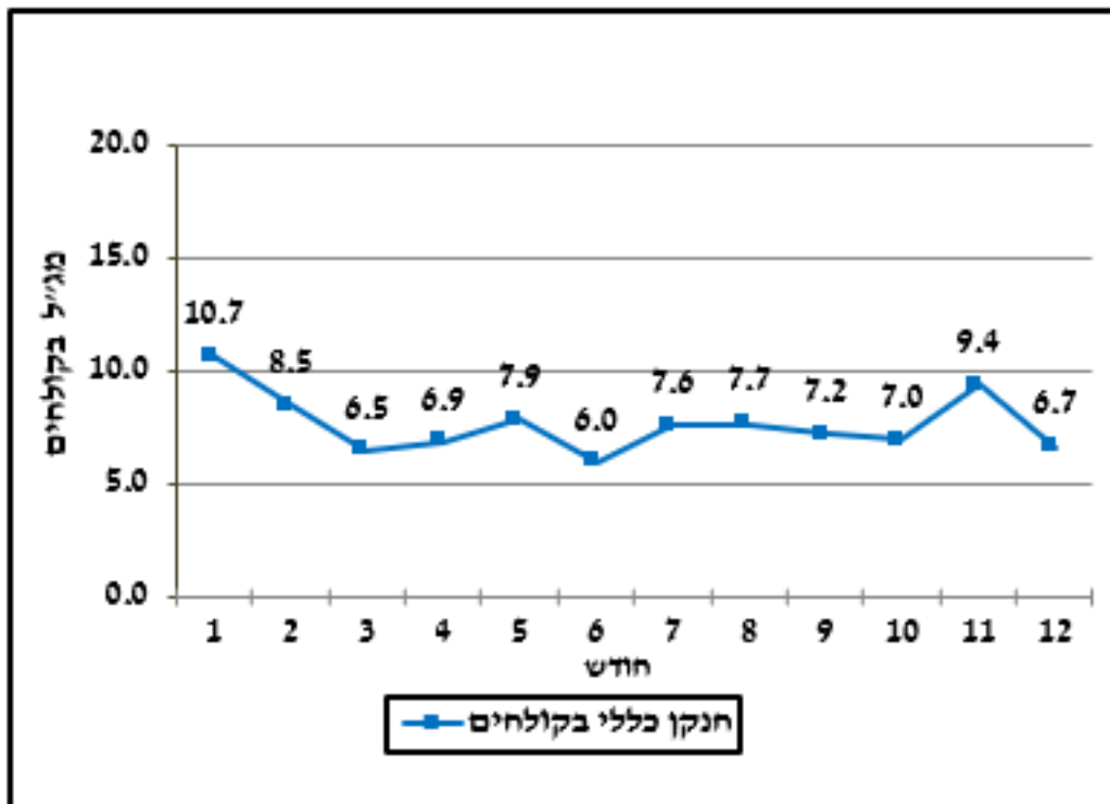
איור 15: ערכי חנקן כללי בקולחים 2023
